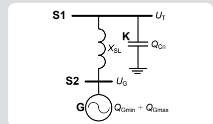
Rys. 6. Schemat modelu kompensatora – model generatorowy z reaktancją i baterią kondensatorów:
