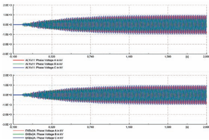
Rys. 7. Napiecia fazowe na koncach wyłączonego toru I linii EKB-ALY
