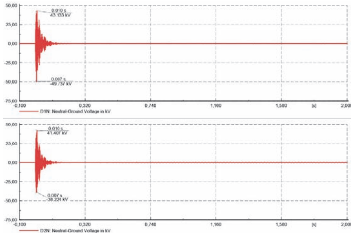
Rys. 5. Napęcia w punkcie gwiazdowym dławików liniowych przyłączonych do szyn stacji Elk Bis
