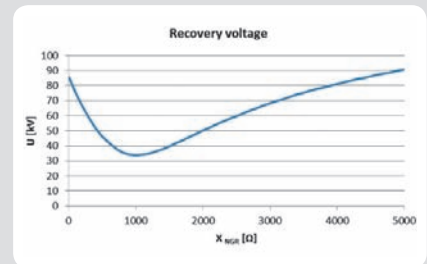
Rys. 9. Napiecia w miejscu zwarcia po jego przeminięciu (ang. recovery voltage ). Zwarcie „łukowe” modelowane rezystancją R = 50 \Omega
