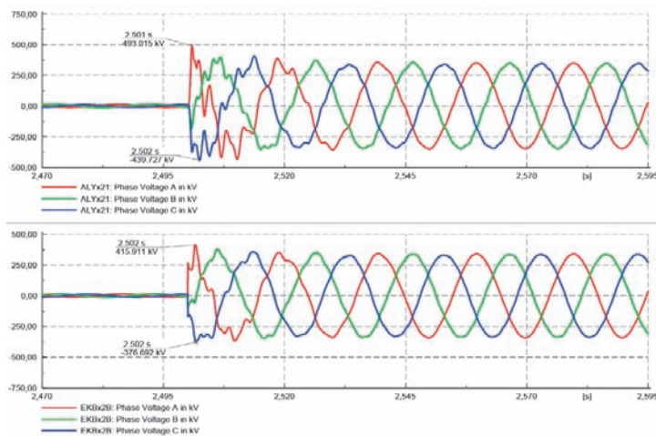
Rys. 6. Napiecia fazowe na koncach toru II linii EKB-ALY
