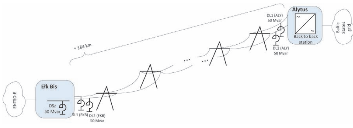
Rys. 1. Schemat poglądowy dwutorowej linii elektroenergetycznej 400 kV Ełk Bis – Alytus
